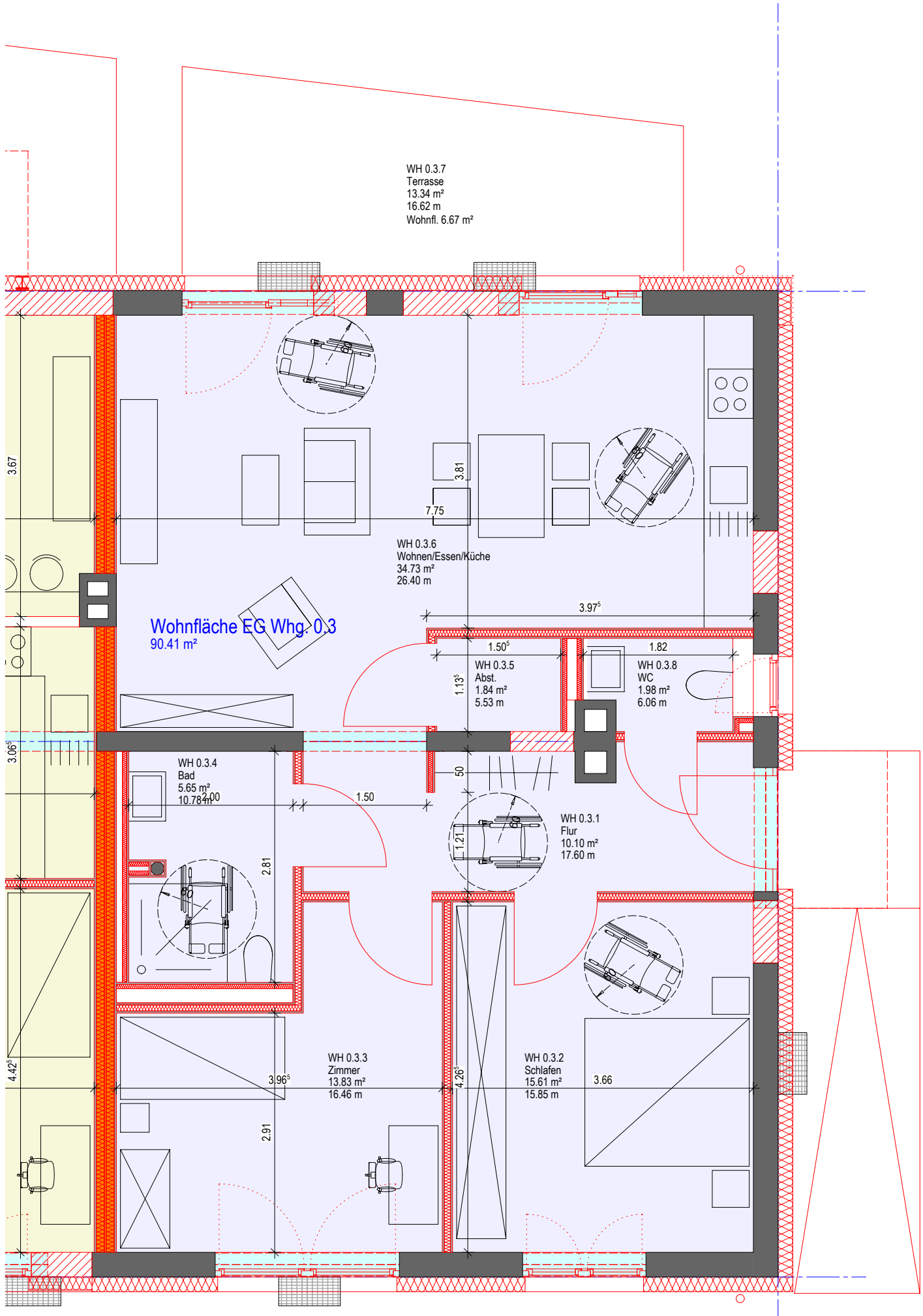
Wohnung EG links 1 : 60
